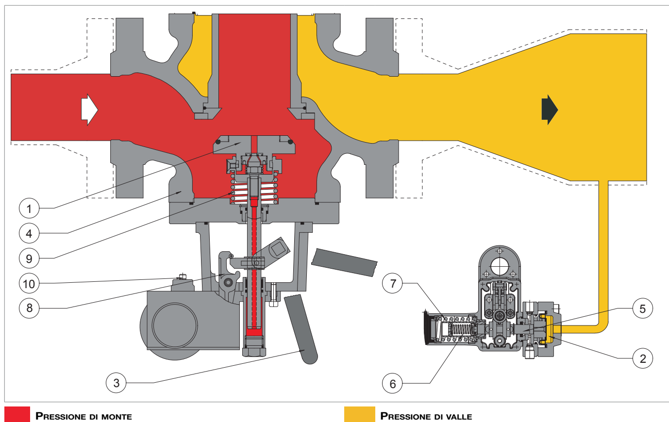
Fig. 4.12. REVAL 182 con valvola di blocco incorporata SB/82
