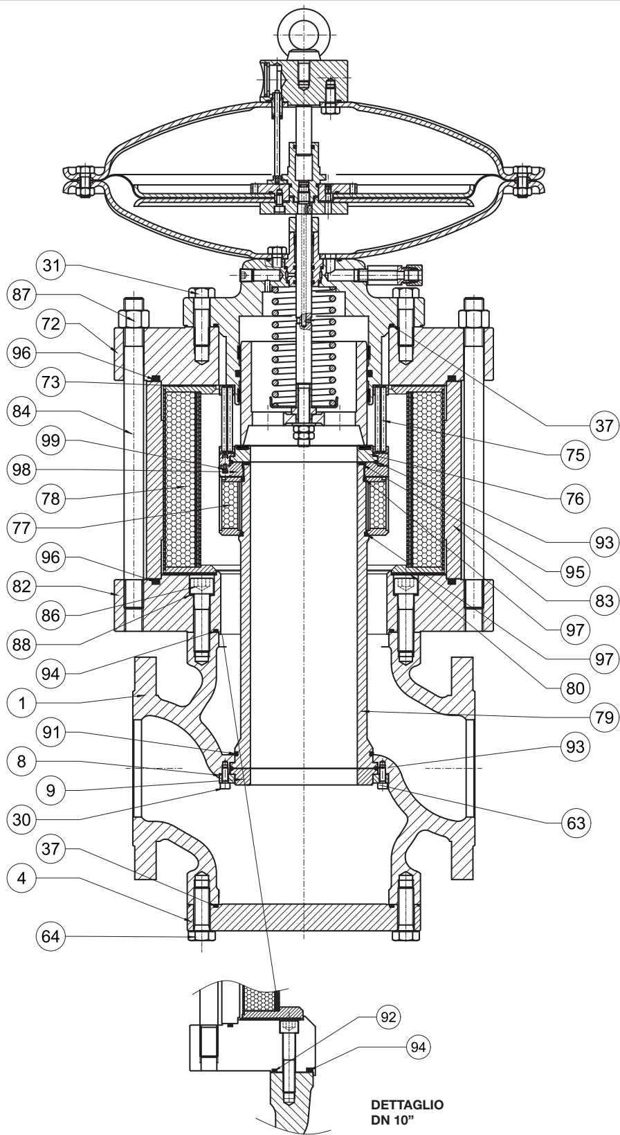
Fig. 9.73. Silenziatore DB/182
