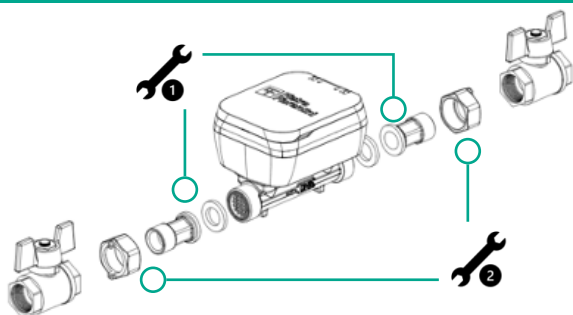
Obr. 1.6. spoje měřiče
