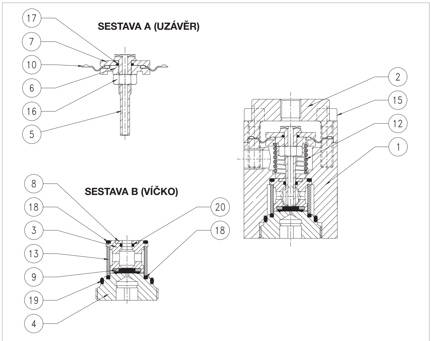
Obr. 9.67. omezovač R14/A
