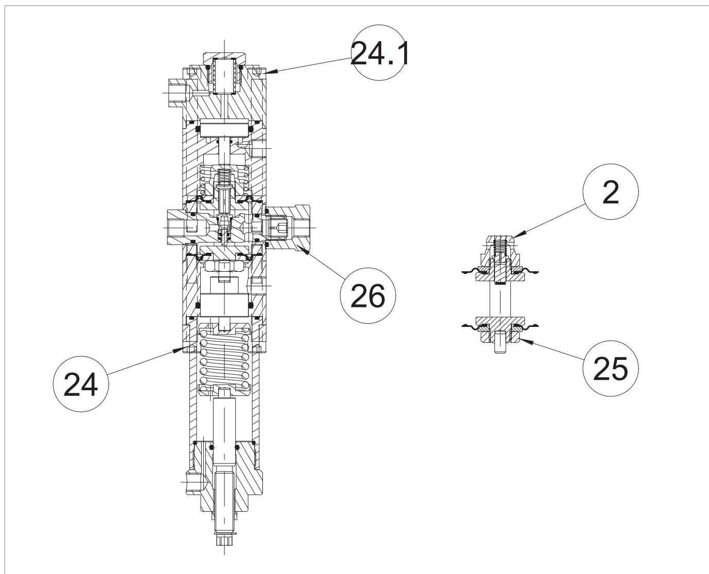
Obr. 9.53. Uťahovací momenty regulátoru R44/SS
