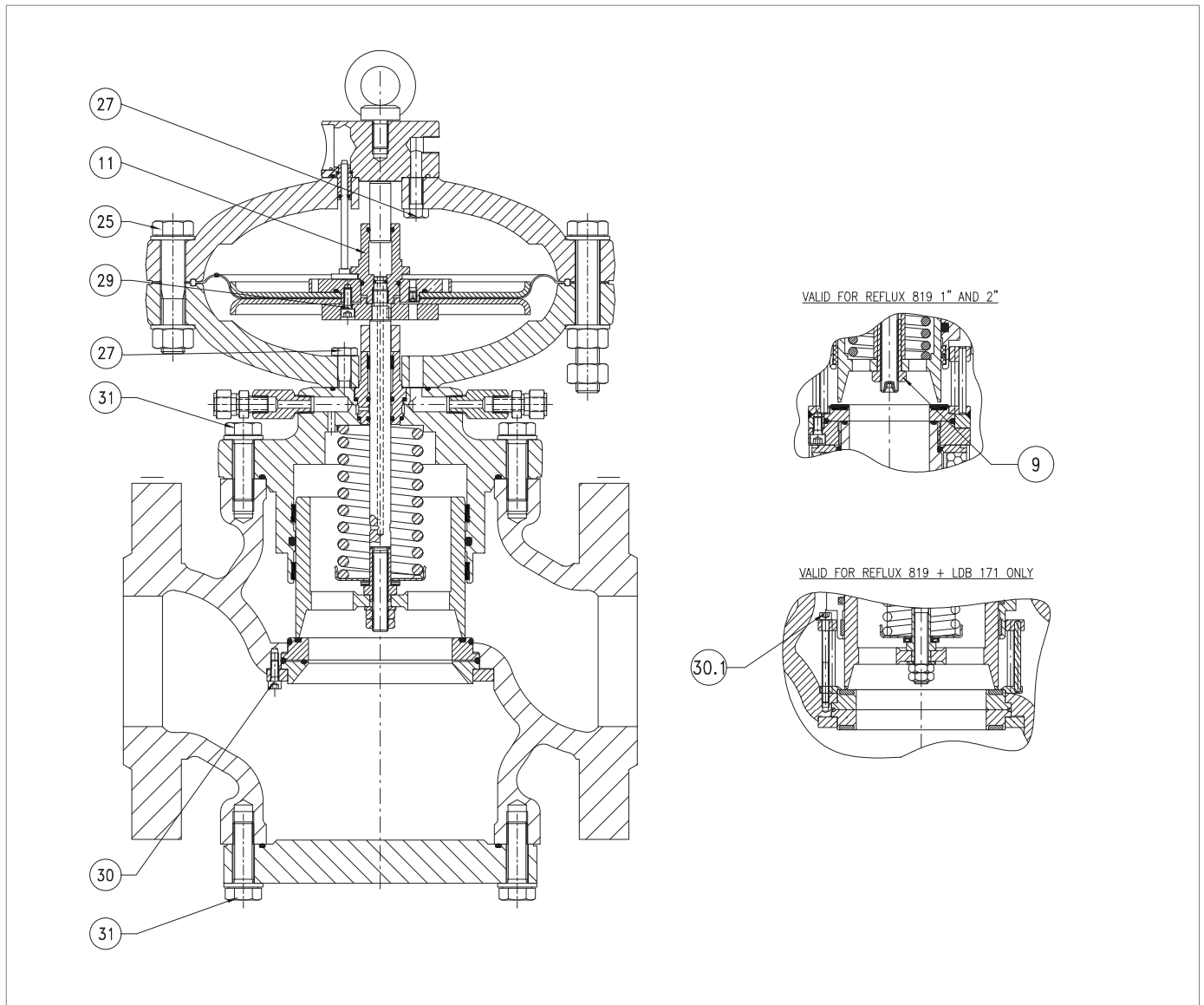
Utahovací momenty REFLUX 819
