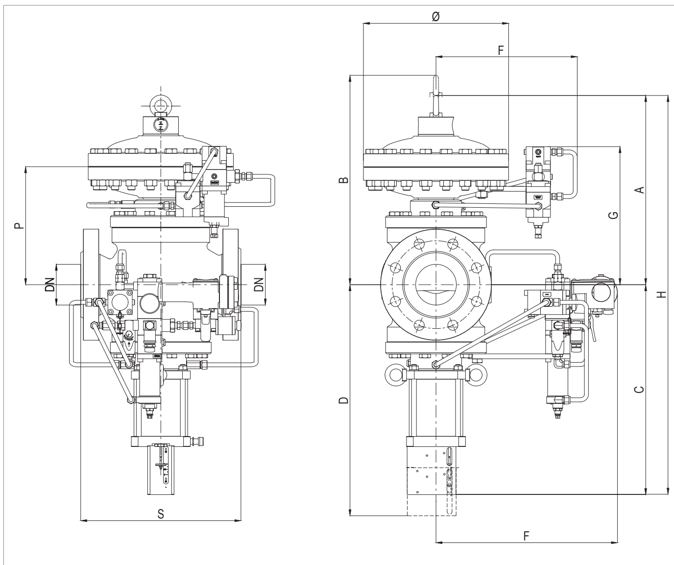
Obr. 5.18. Fyzické vlastnosti REFLUX 819 + HB/97
