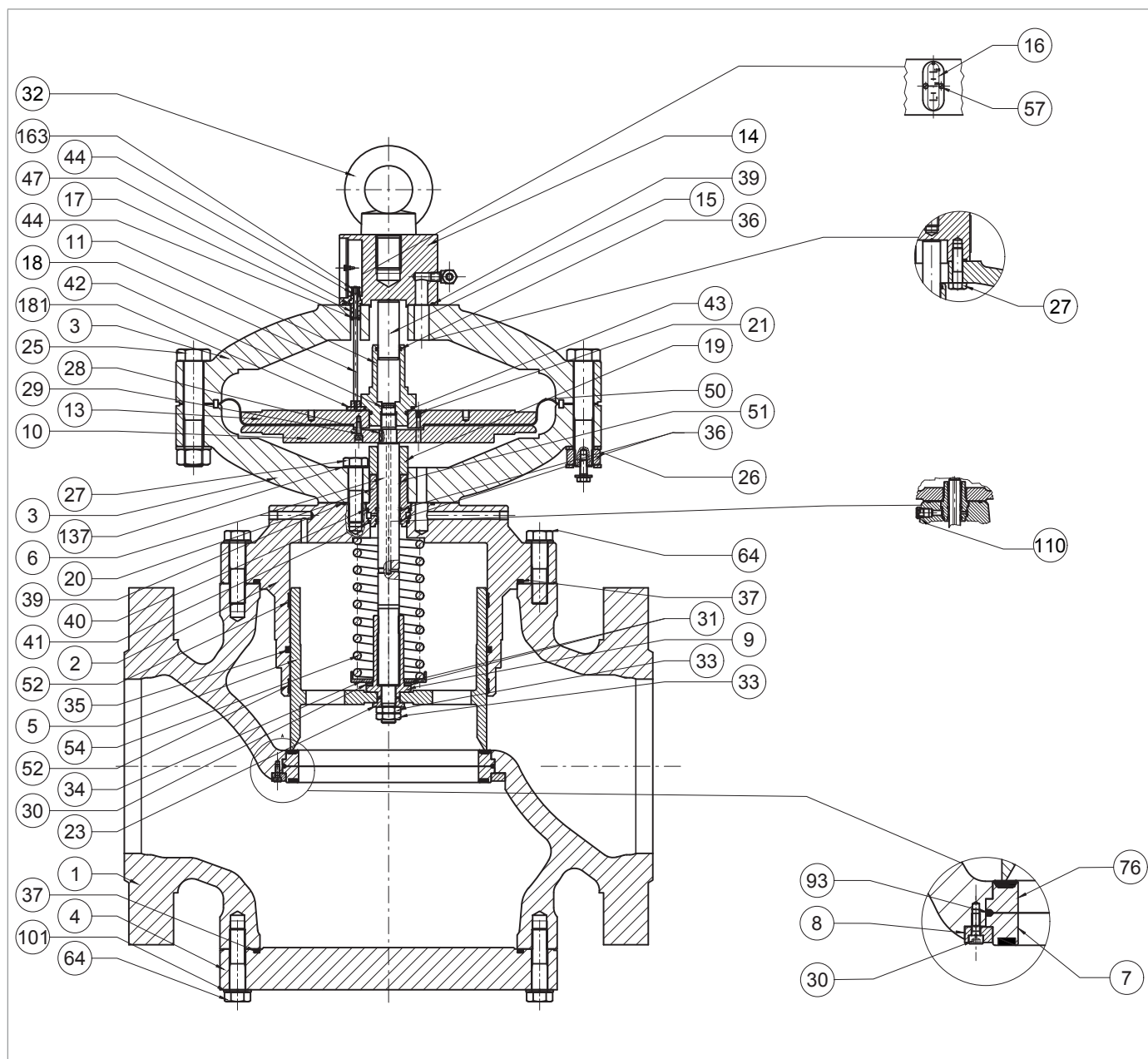
Obr. 9.58. Regulátor REFLUX 819 10"
