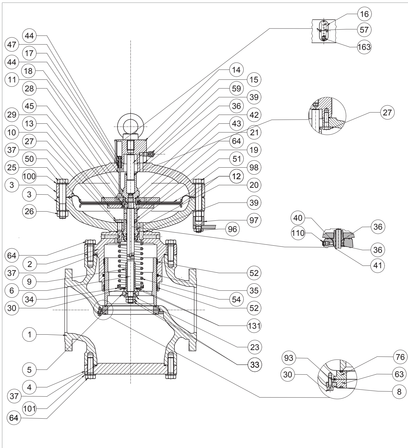
Obr. 9.57. Regulátor REFLUX 819 6" ÷ 8"
