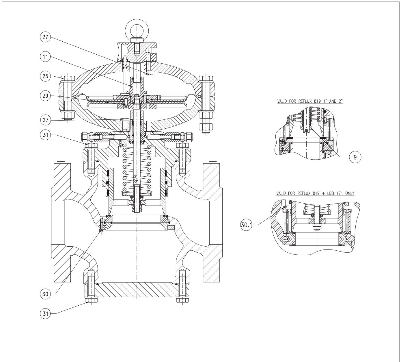
Obr. 9.39. Uťahovací momenty REFLUX 819
